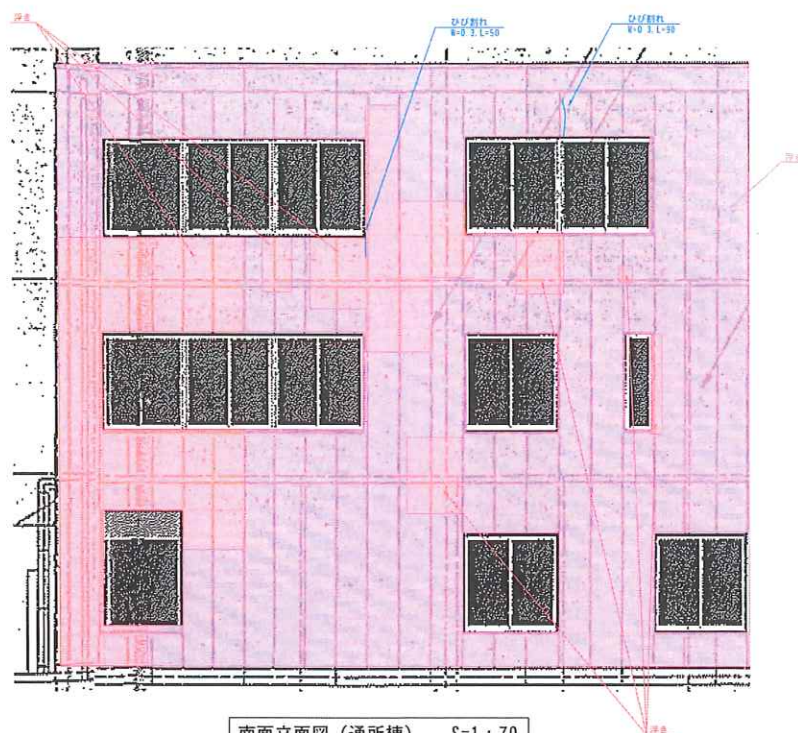
南面立面图 (通所棟) S=1:70
